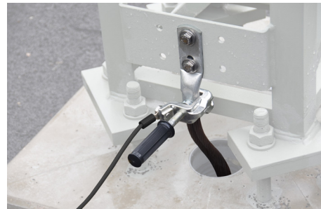
Erdverbindung mit Universalklemme
