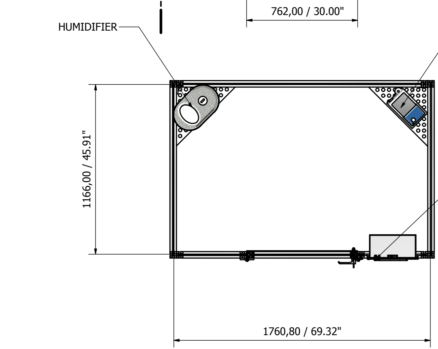
B-B ( 1 : 15 )
