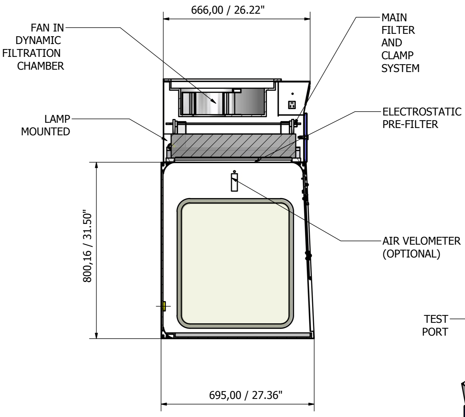
A-A ( 1 : 10 )
