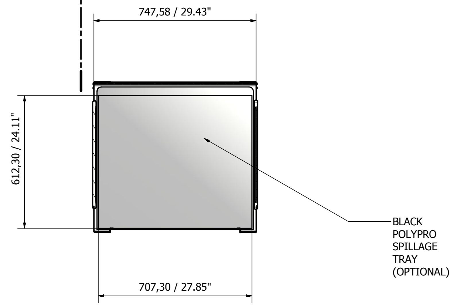
B-B ( 1 : 10 )
